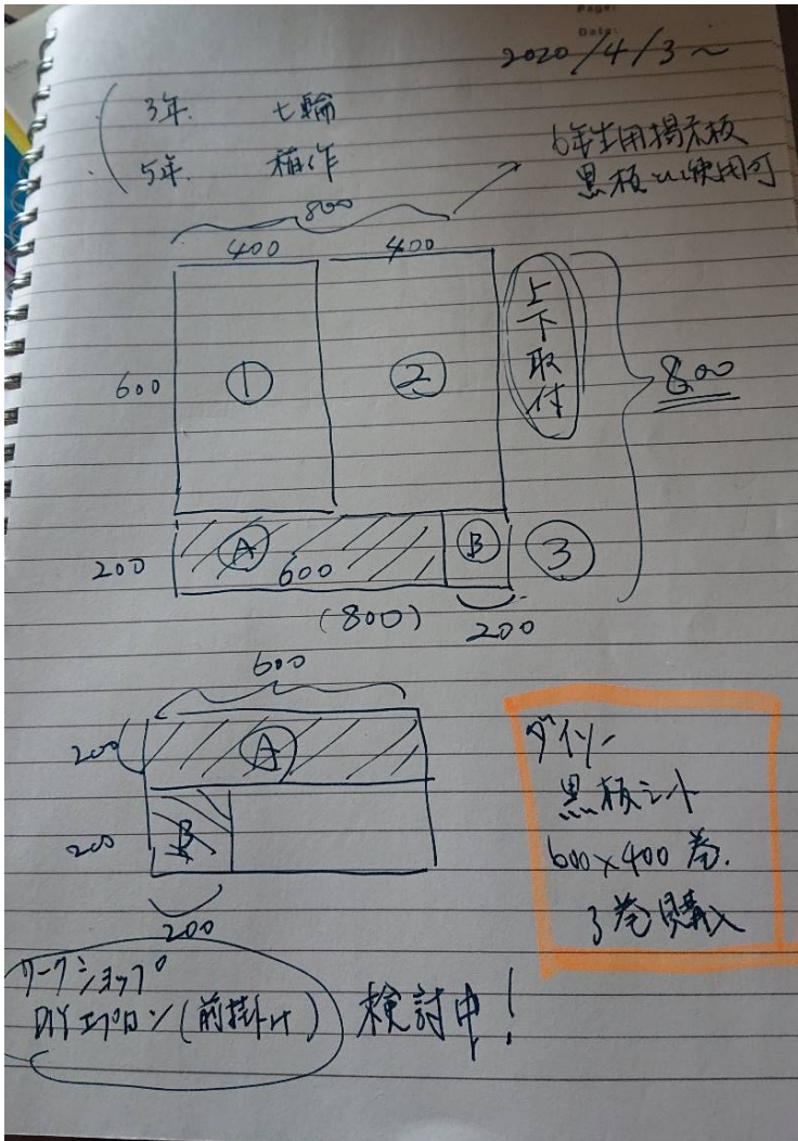
製作構想図↑
