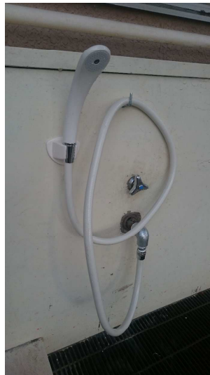
エルボを使って配管サイズをシャワー取付サイズに変換する (3/4B→1/2B 4分)
